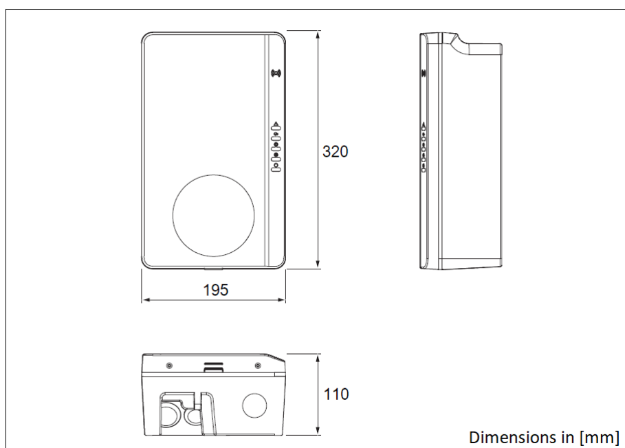
Rozmery: Nabíjačka EV s káblom na nabíjanie EV
