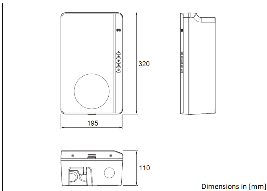
Mál: EV-hleðslutæki með EV-hleðslusnúru
