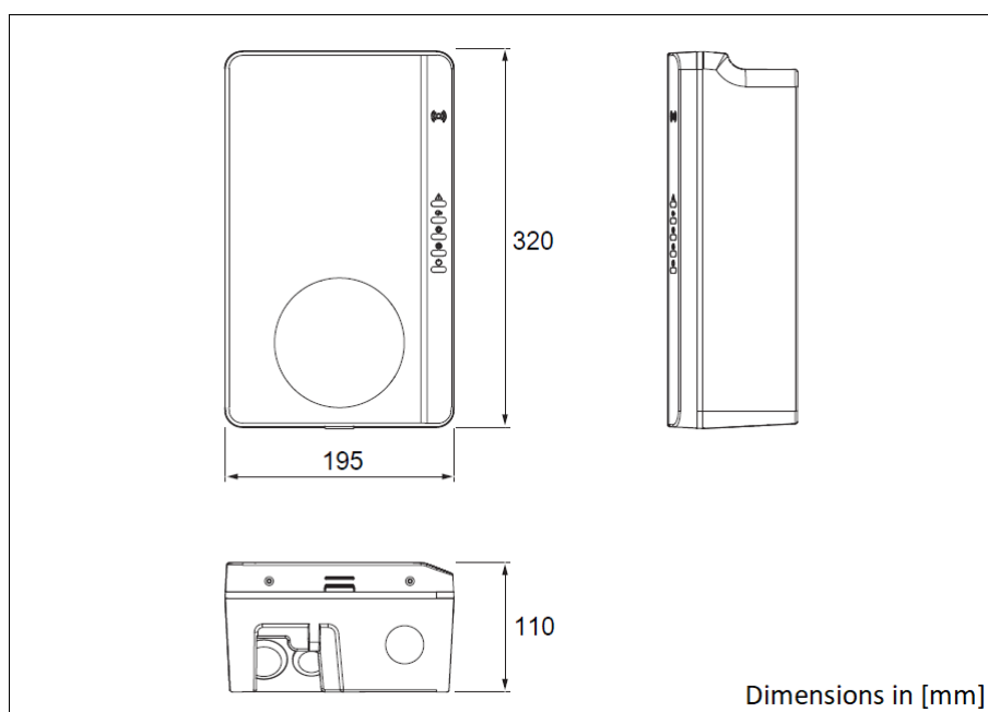
Dimensões: EV Charger com cabo de carregamento VE
