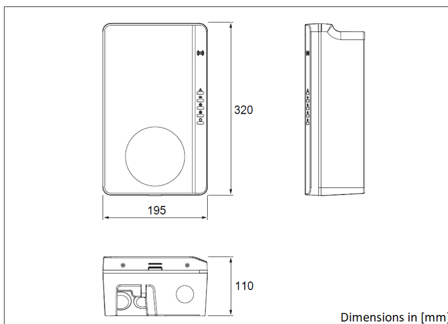
Dimensiuni: Încărcător EV cu cablu de încărcare EV
